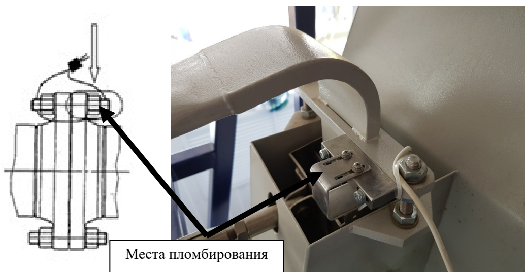
Рисунок 3 – Схема пломбировки от несанкционированного доступа, обозначение места нанесения знаков поверки на фланцевые соединения расходомеров и на оптодатчики положения перегородки устройства переключения потока (при их наличии) установок поверочных УПСЖ-ПРО
